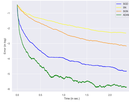
(c) J = 300 - n_{\max} = 19024 (SGD), 687(SN), (d) J = 400 - n_{\max} = 15726 (SGD), 230(SN), 3140(SGN), 20000(ADAM) 633(SGN), 20000(ADAM)
