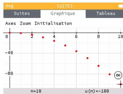
FIGURE 4.3 – Graphique associé à la suite w_n = -n^2
