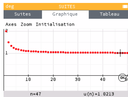
FIGURE 4.1 – Graphique associé à la suite (u_n)_{n \geq 0}
