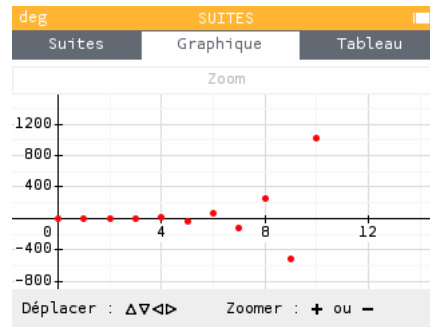
FIGURE 4.4 – Graphique associé à la suite (t_n)_{n \geq 0}
