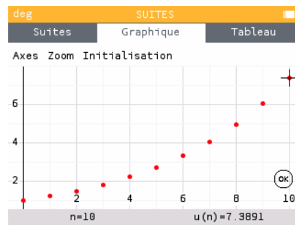
FIGURE 4.2 – Graphique associé à la suite v_n = e^{0,2n}
