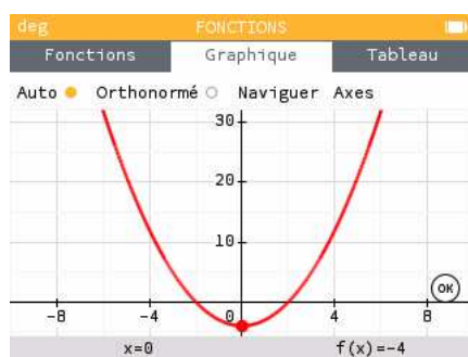
FIGURE 9.1: Représentation de y = x^2 - 4
